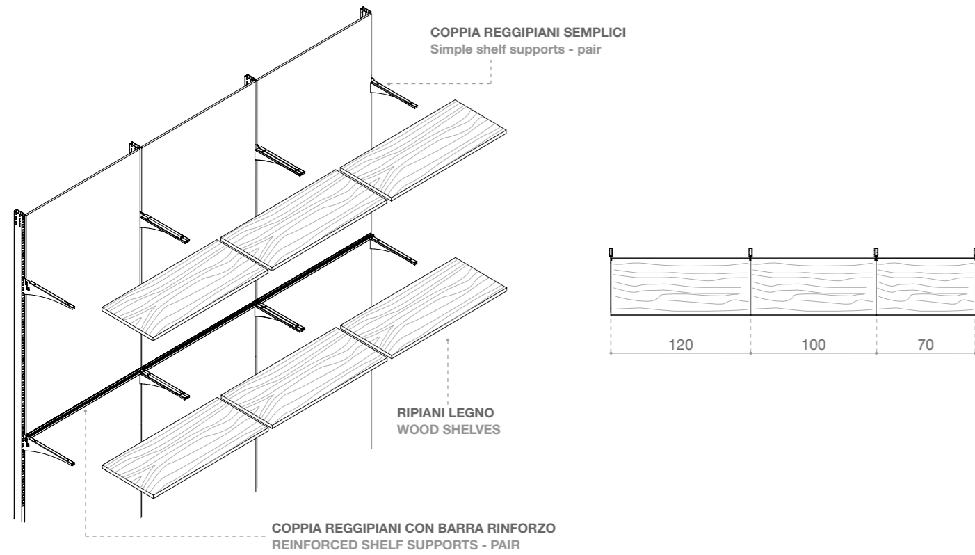
CARICHI PER REGGIPIANI SEMPLICI LOADS FOR SIMPLE SHELF SUPPORTS
