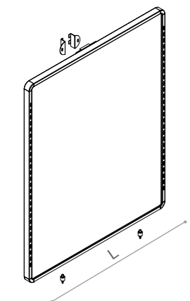
64 Kit pannello cremagliere verticali testata gondola su ripiano base Gondola head lateral uprights panel set on base shelf materiali: materials: B00 B01 B02 B03 B04
