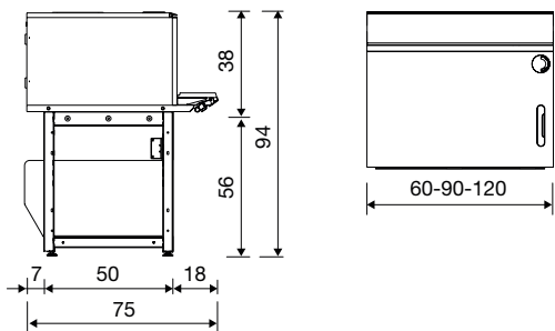
Volume cassettiera diritto Straight drawers element
