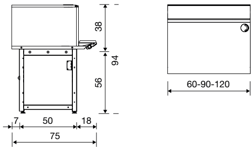
Volume antitaccheggio diritto Straight anti-theft element
