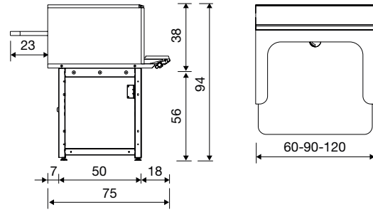
Volume angolare Corner element
